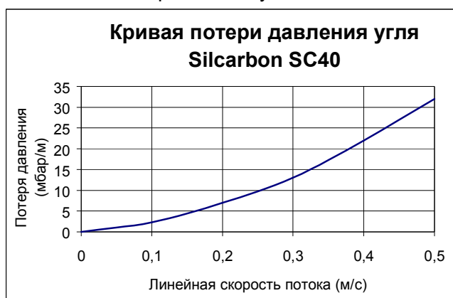
Рисунок 1: Кривая потери давления угля Silcarbon SC40.
